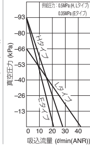
流量特性
