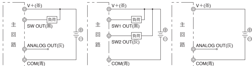
アナログ出力付圧力センサ(-NA)結線図 2点スイッチ出力付圧力センサ(-NW)結線図 アナログ1点出力圧力センサ(-A)結線図
