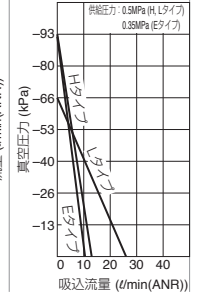
流量特性
