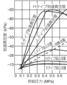
真空特性
