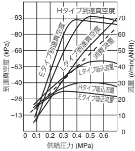
真空特性
